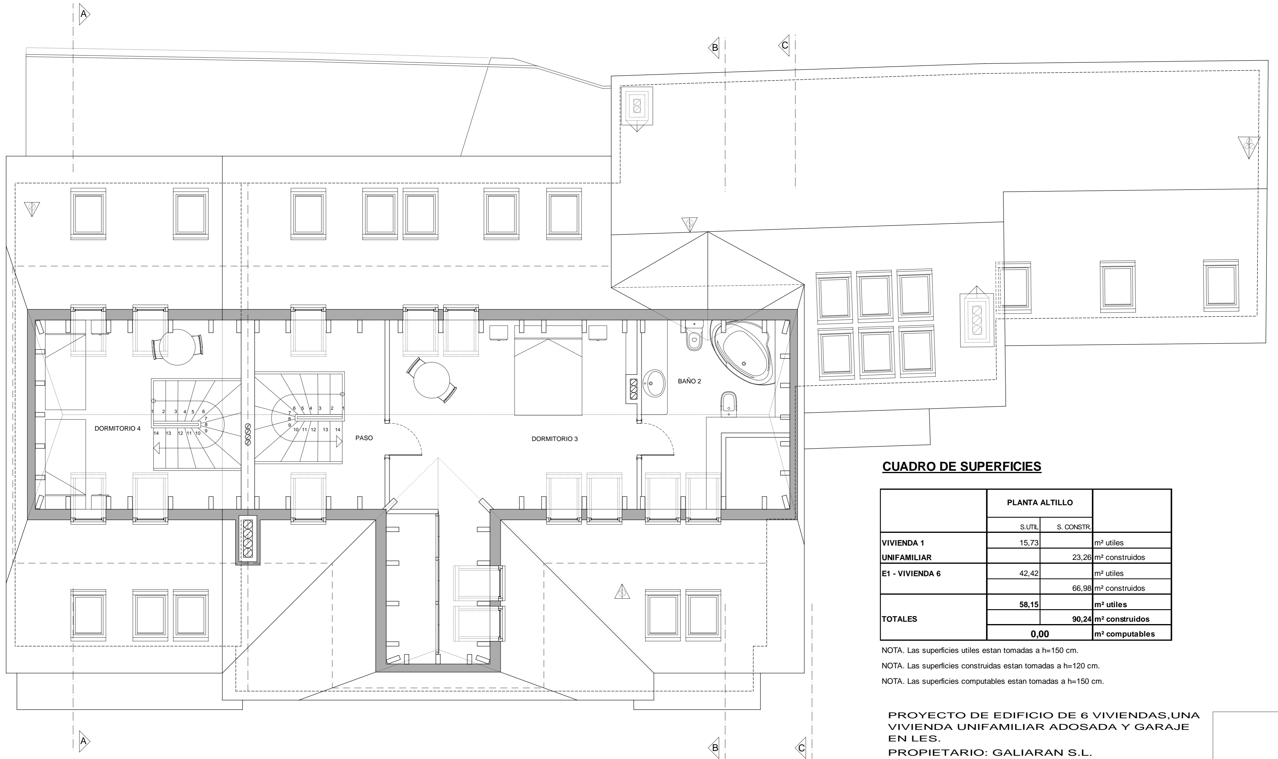
PLANTA ALTILLO
