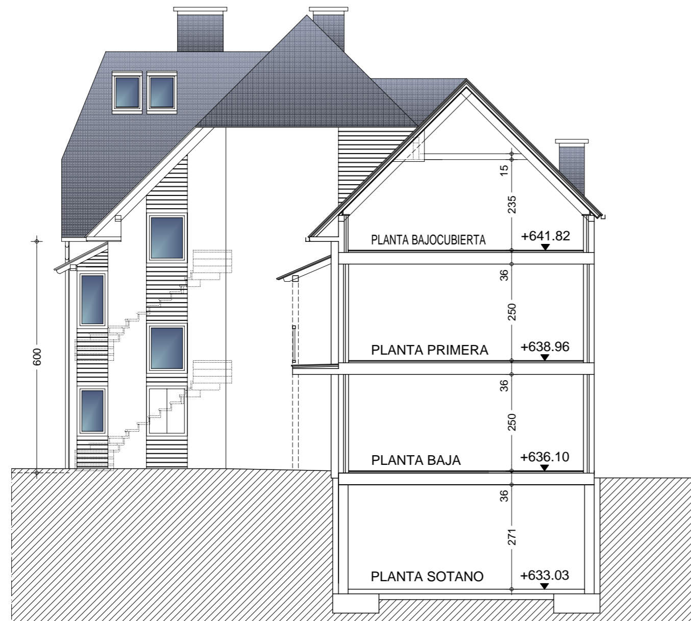
SECCION C-C
