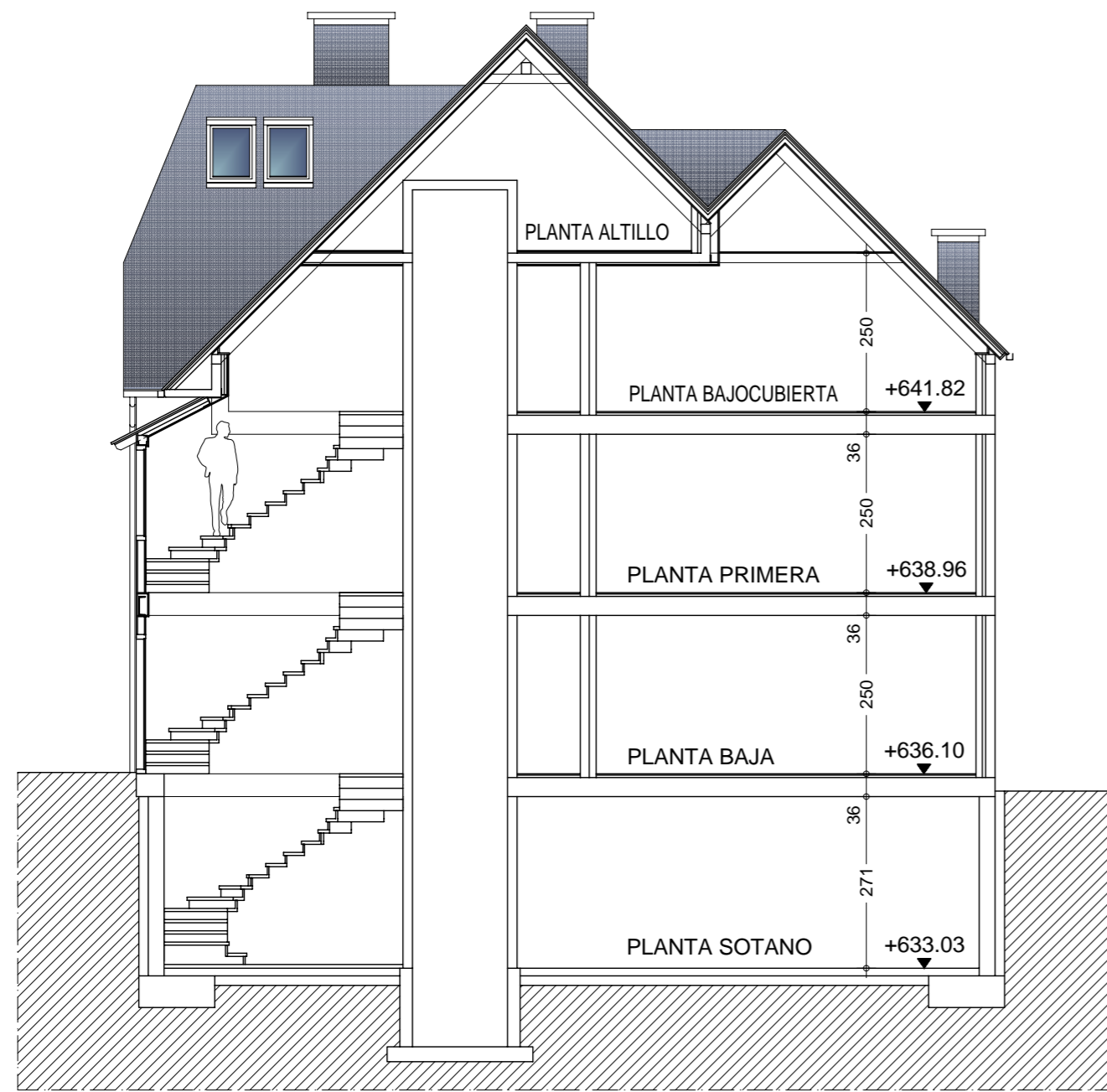
SECCION B-B
